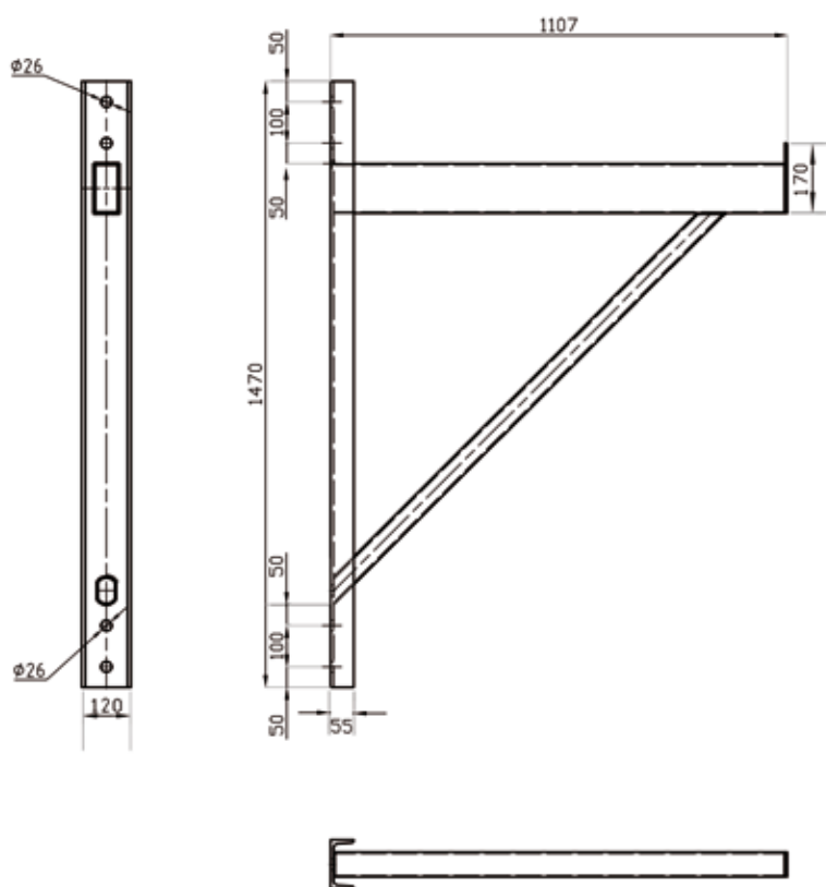
Maatvoering muurconsole licht artnr. 0703/960
