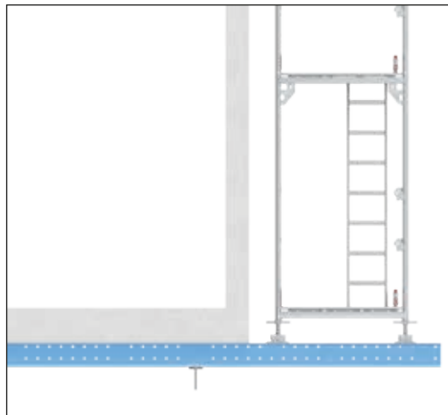
Console amarrée à la dalle
