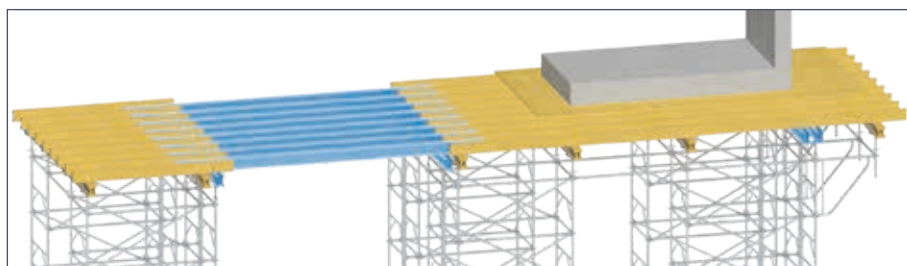
Combinaison de TwixBeam et de supports H-20 au même niveau.
