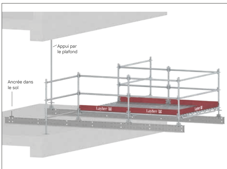
Plate-forme en porte-à-faux - ancrée dans le sol ou appuyée par la dalle de plancher.
