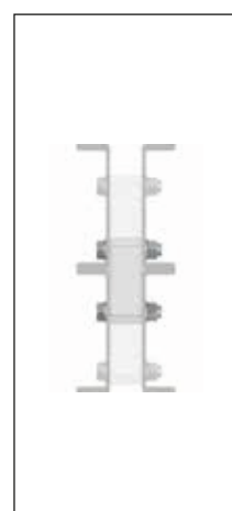
Poutres placées l'une sur l'autre bloquées par colliers (gauche) ou avec un espaceur (droite)
