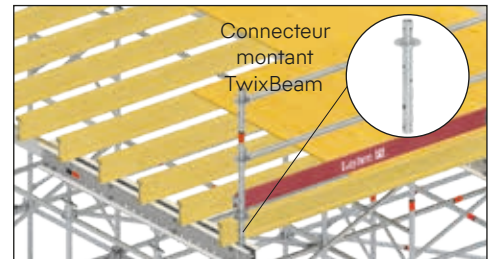
Protection des bords intégrée avec le connecteur montant TwixBeam
