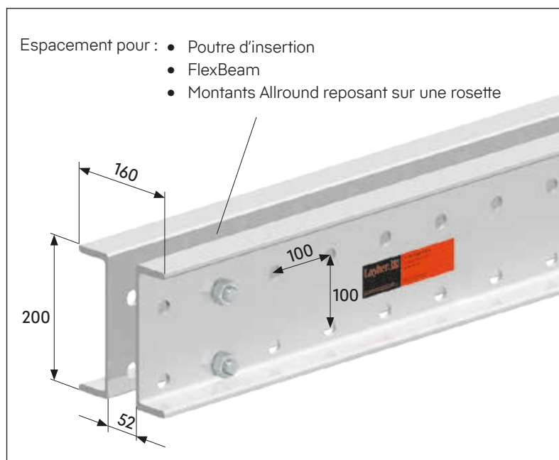
Dimensions du poutre TwixBeam en aluminium de 0,80 à 6,60 m de longueur
