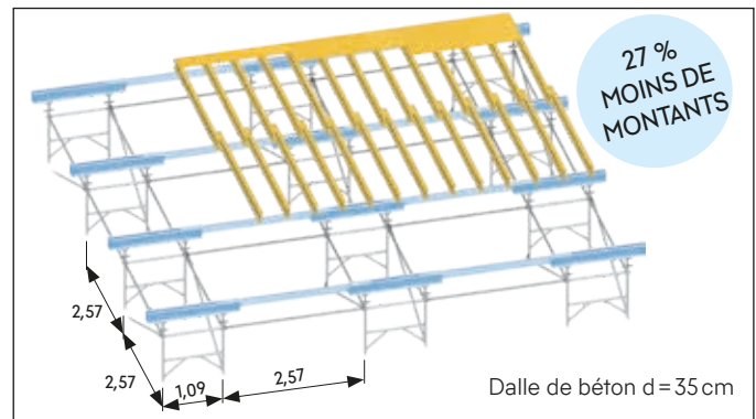
TwixBeam. Structure allongée. Surface par tour de support 18,8 m 2 Charge standard d'environ 51 kN → Nombre de montants env. - 27 %
