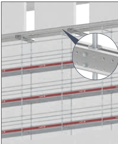
Échafaudage de soutien suspendu
