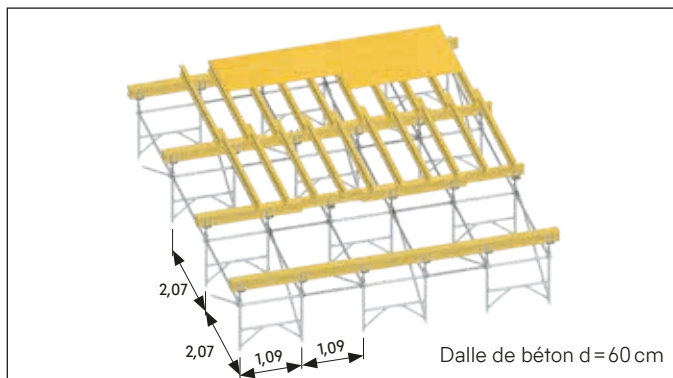
H-20-Double support en bois. Structure compacte. Surface par tour de support 9,0 m 2 . Charge standard d'environ 40 kN
