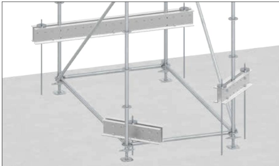
Tour amarée au sol.
