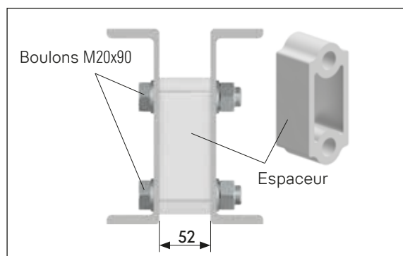
La poutre TwixBeam en coupe transversale
