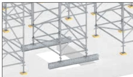
Pontage dans la zone de base
