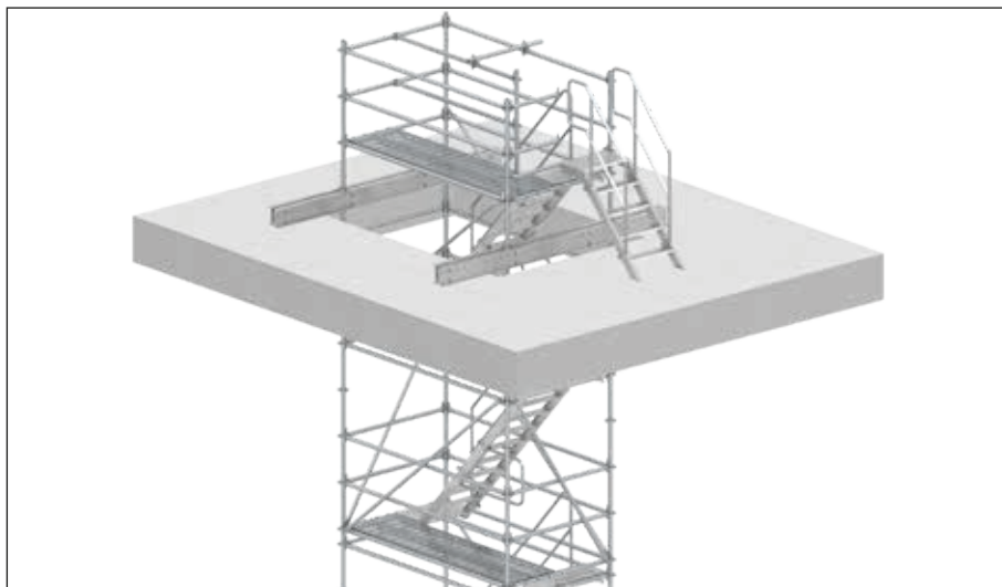
Tour d'escaliers suspendue (volées modulaires Allround)
