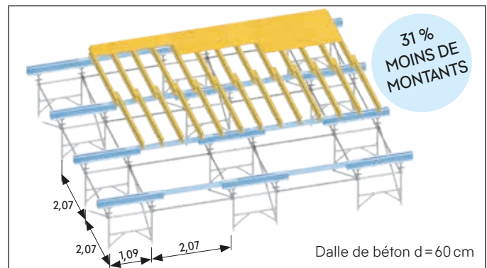
TwixBeam. Structure allongée. Surface par tour de support 13,1 m 2 Charge standard d'environ 58 kN → Nombre de montants env. - 31 %
