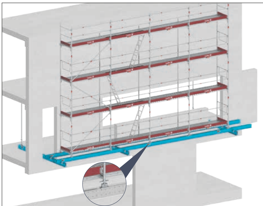
Echafaudage de soutien surélevé - construction TwixBeam montée comme une grille de poutrelles - soutenu par la surface du sol.
