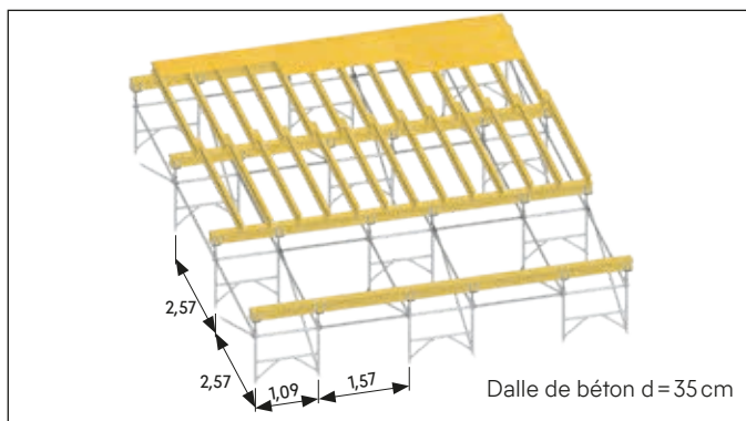
H-20-Double support en bois. Structure compacte. Surface par tour de support 13,7 m 2 . Charge standard d'environ 37 kN
